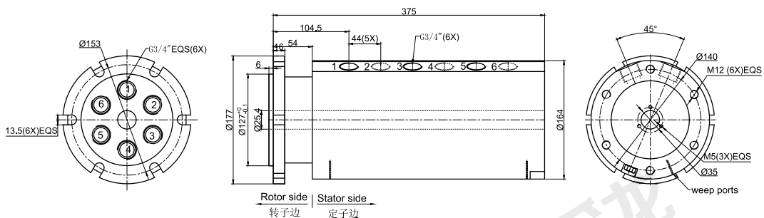
MVH66 (大流量旋转接头) 尺寸图
