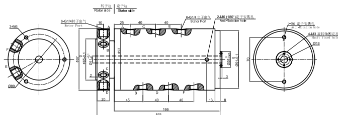
MQ600F-03 尺寸图
