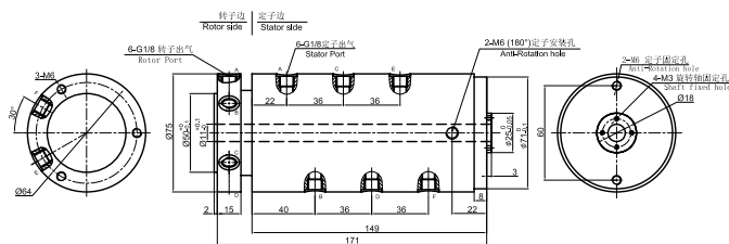
MQ600F-02 尺寸图
