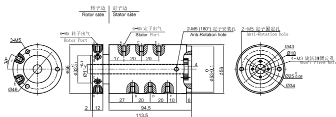
MQ600F-01 尺寸图
