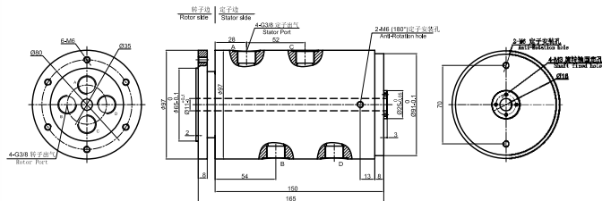
MQ400-04 尺寸图
