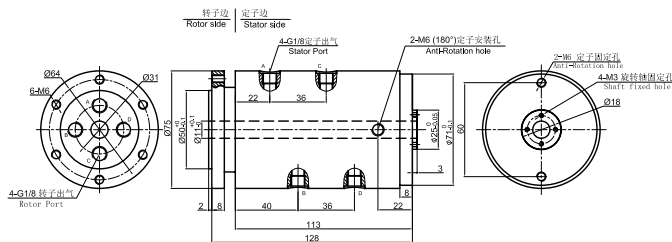
MQ400-02 尺寸图
