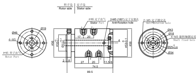
MQ400-01 尺寸图
