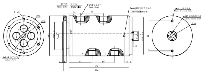
MQ400-05 尺寸图
