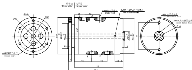
MQ400-03 尺寸图
